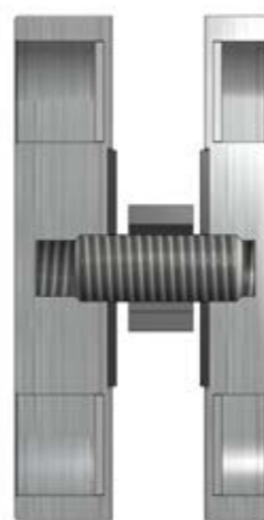
Schnittansicht der GM.6605, Standardlieferung Section view of GM.6605, standard version
