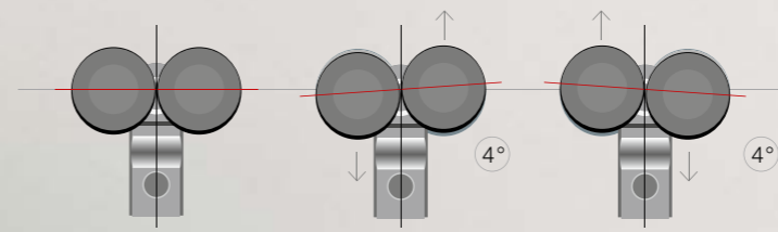
Flexible Rollenlagerung sichert eine gleichmäßige Kräfteverteilung Flexible roller bearings ensure an even distribution of forces
