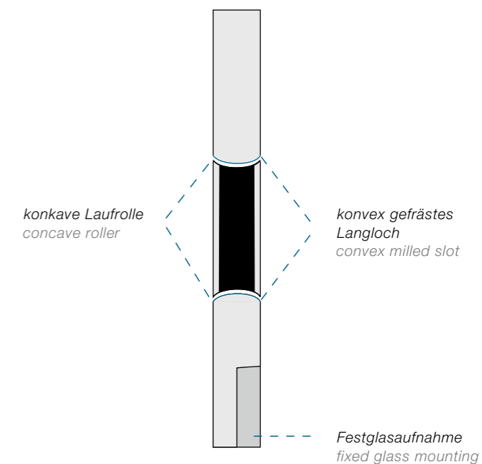
Querschnitt Laufschiene/Laufrolle Cross section of track/track roller
