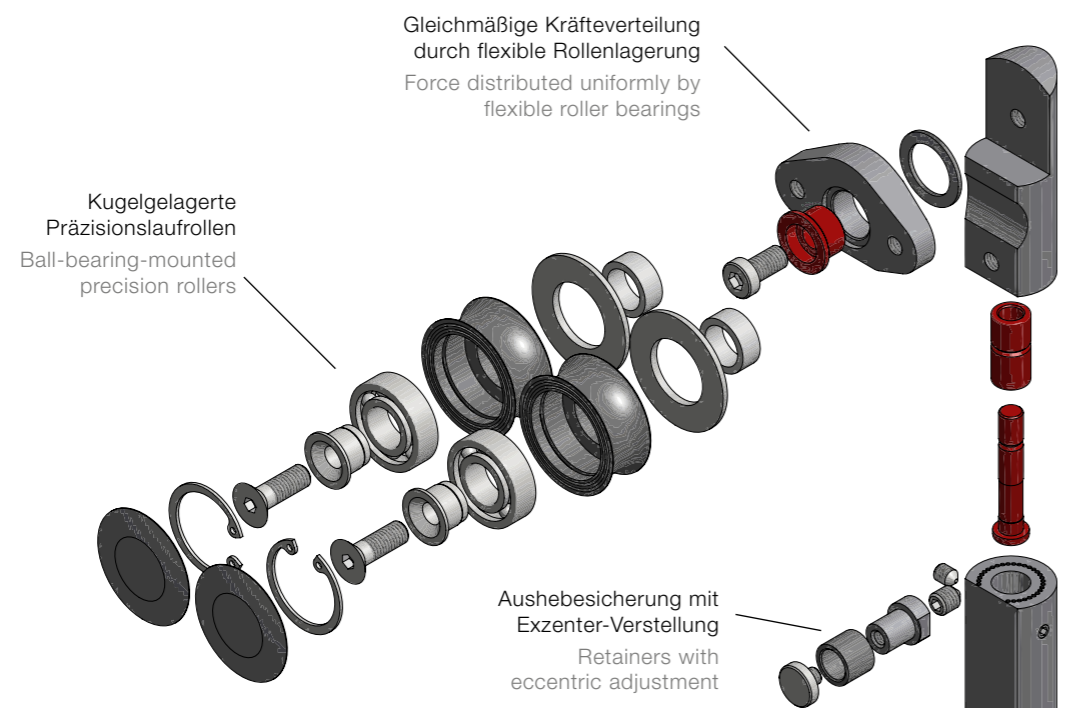
Anordnungsplan 3D Rollwagen System Vario Modell 2013
